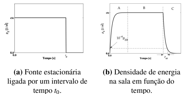
Figura 2: Comportamento de um fonte sonora constante e densidade de energia em campo difuso (extraído de Brandão [4]).
