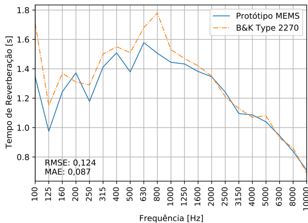
Figura 9: Tempo de reverberação da sala de aula medido com o protótipo e com o B&K Type 2270.
