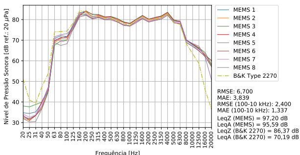
Figura 10: Níveis de pressão sonora medidos com oito microfones MEMS e com o B&K Type 2270, para o sinal de ruído branco.
