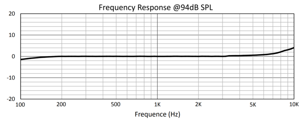
Figura 4: Curva de sensibilidade do MEMS [13].
