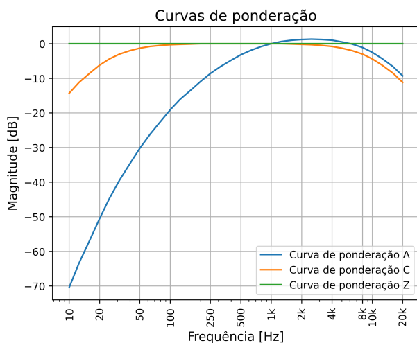
Figura 1: Curvas de ponderação A, C e Z conforme a norma IEC 61672-2013 [6].
