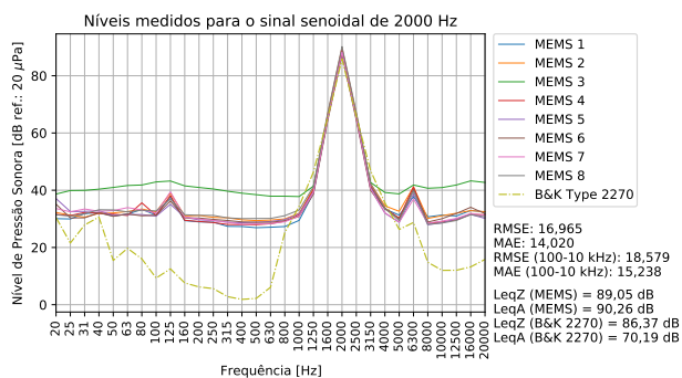
Figura 16: Níveis de pressão sonora medidos com oito microfones MEMS e com o B&K Type 2270, para o sinal de 2000 Hz.
