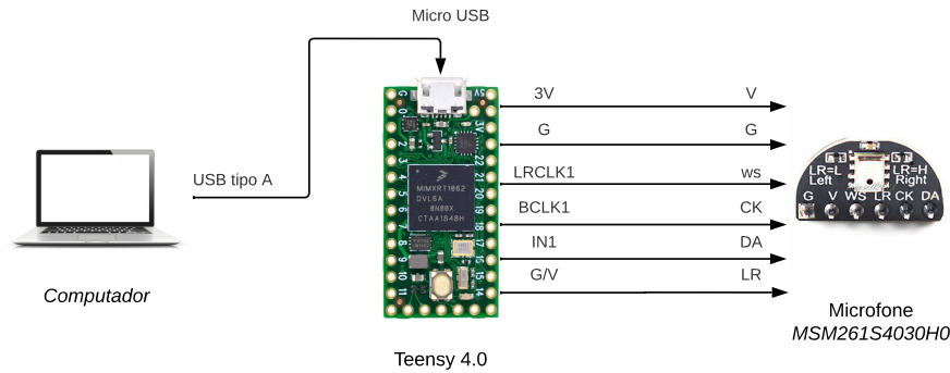
Figura 3: Diagrama das conexões do microfone MEMS com o computador.
