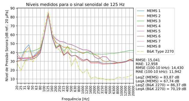
Figura 13: Níveis de pressão sonora medidos com oito microfones MEMS e com o B&K Type 2270, para o sinal de 125 Hz.
