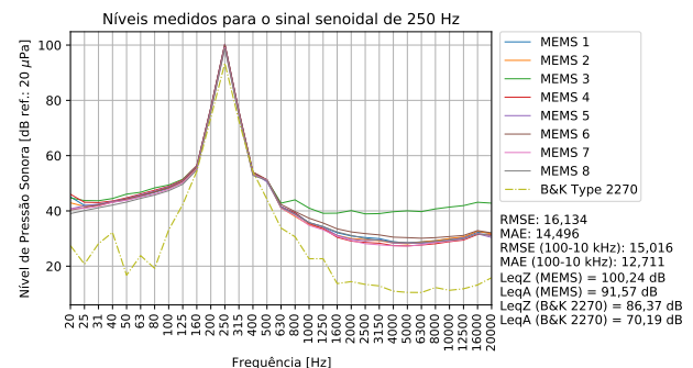
Figura 14: Níveis de pressão sonora medidos com oito microfones MEMS e com o B&K Type 2270, para o sinal de 250 Hz.
