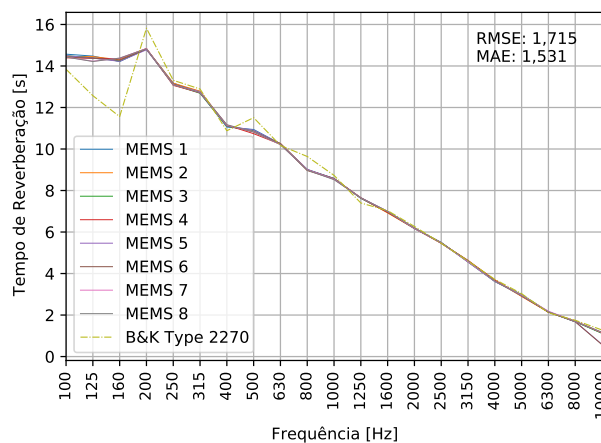
Figura 8: Tempo de reverberação da câmara reverberante medido com oito microfones MEMS e com o B&K Type 2270.
