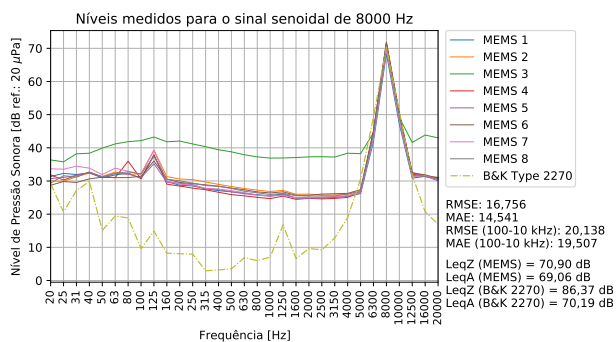
Figura 18: Níveis de pressão sonora medidos com oito microfones MEMS e com o B&K Type 2270, para o sinal de 8000 Hz.
