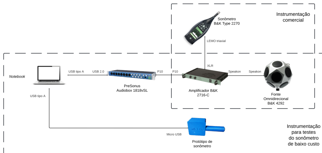
Figura 6: Cadeia de medição de tempo de reverberação.
