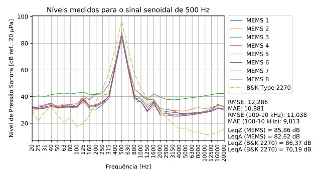
Figura 15: Níveis de pressão sonora medidos com oito microfones MEMS e com o B&K Type 2270, para o sinal de 500 Hz.
