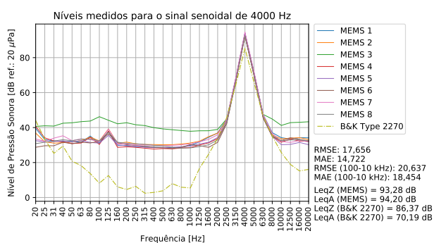
Figura 17: Níveis de pressão sonora medidos com oito microfones MEMS e com o B&K Type 2270, para o sinal de 4000 Hz.
