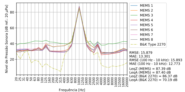
Figura 11: Níveis de pressão sonora medidos com oito microfones MEMS e com o B&K Type 2270, para o sinal em 1000 Hz.
